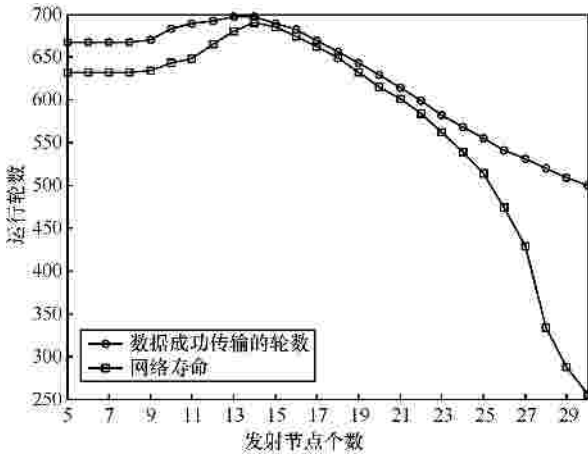
图 8 数据成功传输的轮数及网络寿命
