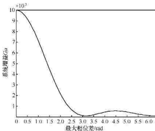
图 2 系统增益随最大相位差 j_{\max} 变化时的性能
