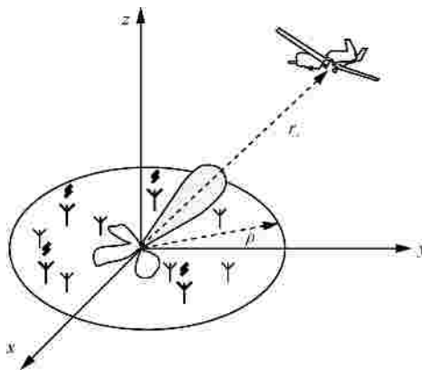
图 1 波束成形示意
